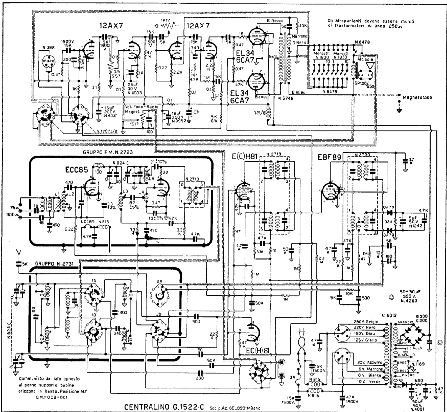
Vista posteriore del centralino G 1522-C
